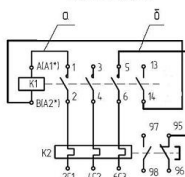
Схема подключения
