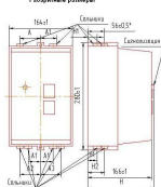
Габаритные размеры
