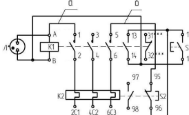
Схема подключения
