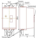
Габаритные размеры
