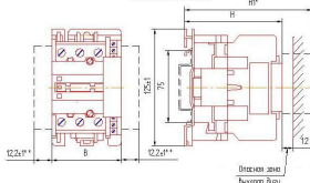
Габаритные размеры
