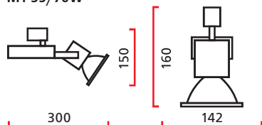
MT 35/70W
