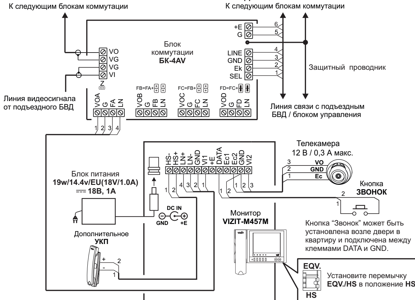
Рисунок 4 - Монитор VIZIT-M457M с дополнительными телекамерой, УКП и кнопкой "Звонок" в составе многоабонентского (подъездного) видеодомофона
