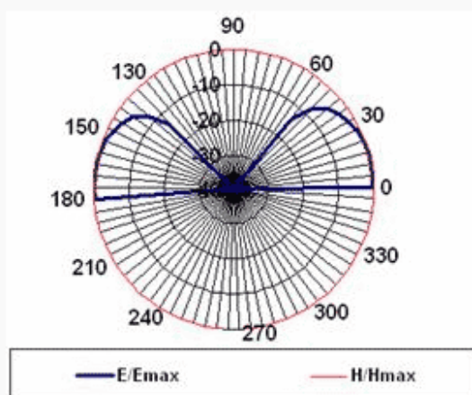
Диаграмма направленности антенны "Шайба" в вертикальной и горизонтальной плоскостях
