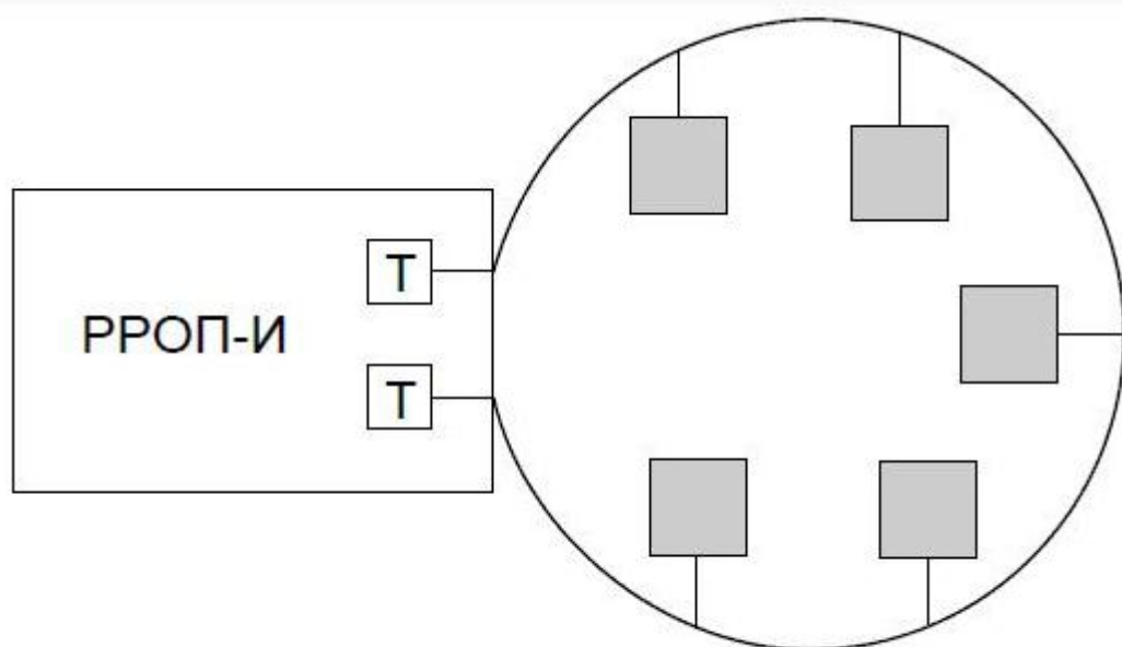
Топология кольцо с использованием двух сетевых интерфейсов РРОП-И
