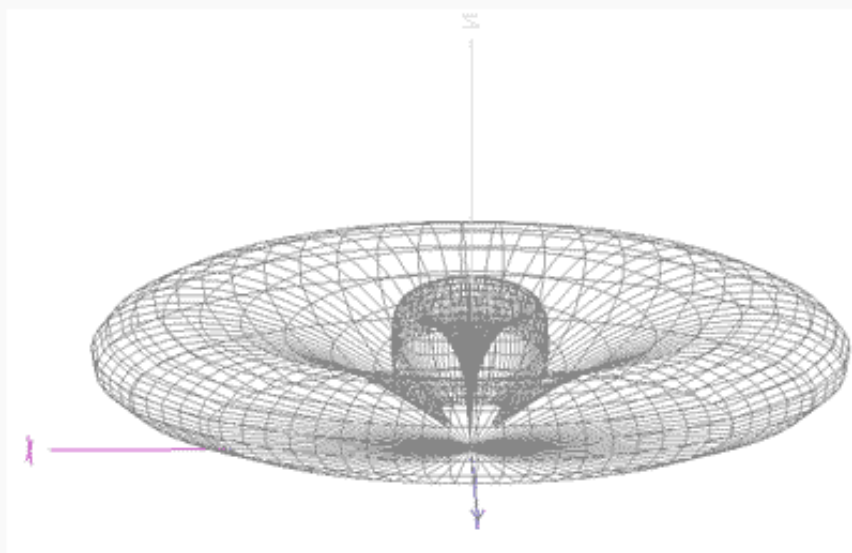
Типовая диаграмма направленности коллинеарной антенны
