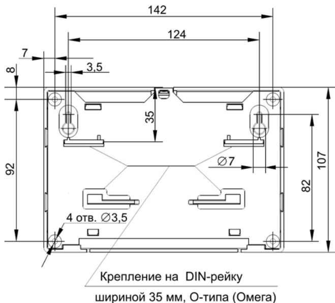
Рисунок 3. Установочные размеры «ПИ-ГР»
