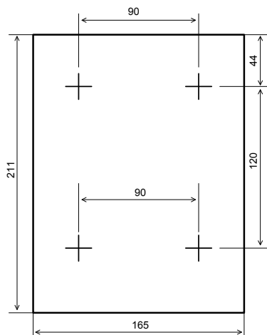
Рисунок 2. Габаритно-установочные размеры
