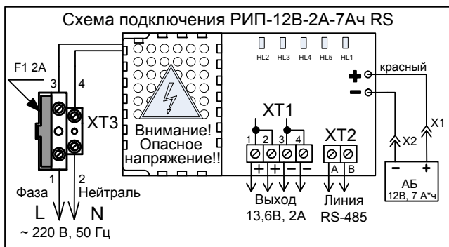
Рисунок 3. Схема подключения «РИП-12В-2А-7Ач RS»
