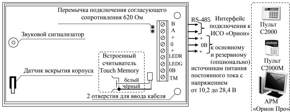
Рисунок 3. Схема внешних соединений блока
