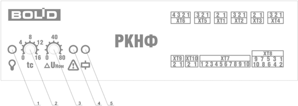
Рисунок 3. Лицевая панель РКНФ
