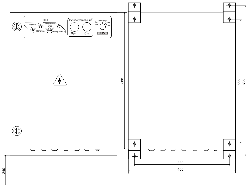
Рисунок 6. Габаритные и установочные размеры шкафа
