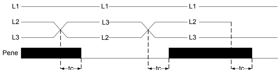
Рисунок 4. Контроль порядка чередования и обрыва фаз
