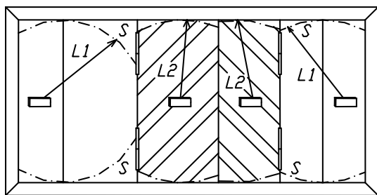
Рисунок 6. Защита немонолитной констр. ( S<0,1\text{м}^2 , L1<L2 )
