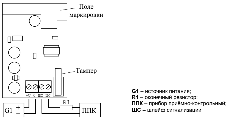
Рисунок 1. Схема подключения извещателя
