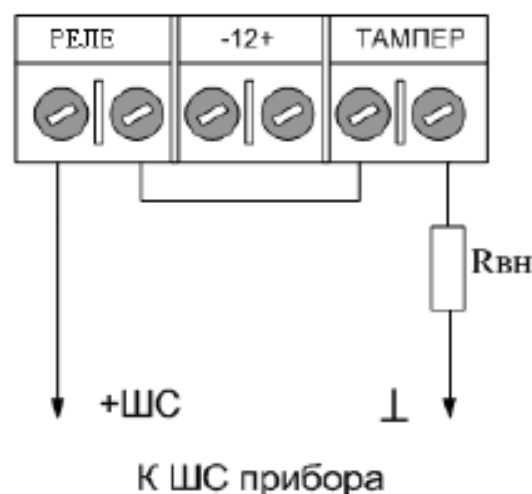
Рисунок 1 – Схема подключения извещателя
