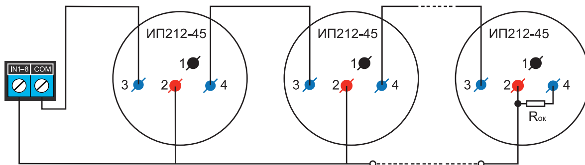
Рисунок 3. Схема подключения ИП212-45 к пожарному входу NV 8804 только с оконечным резистором
