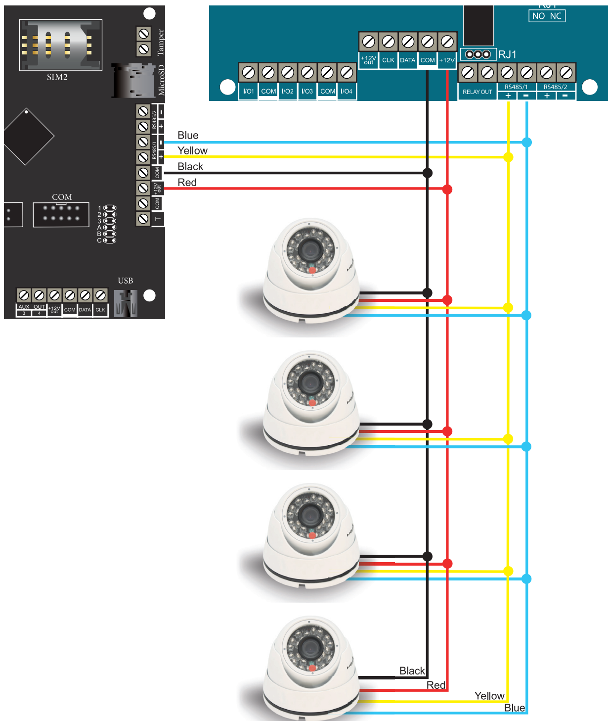
Рисунок 5. Подключение камер NV DOM 485-28IR к NV 8500 и NV 8804
