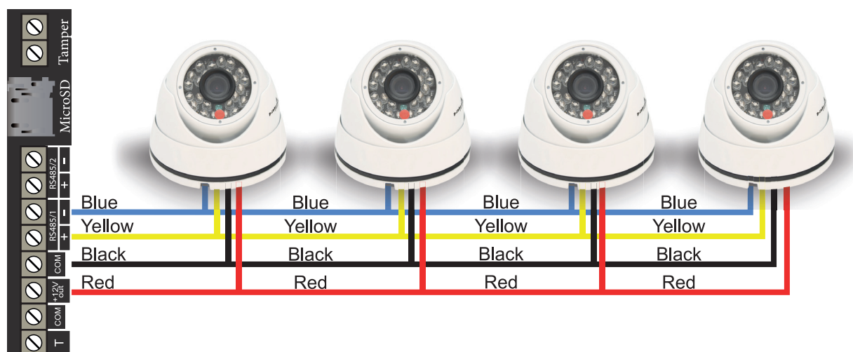
Рисунок 8. Подключение камер NV DOM 485-28IR к NV 8804
