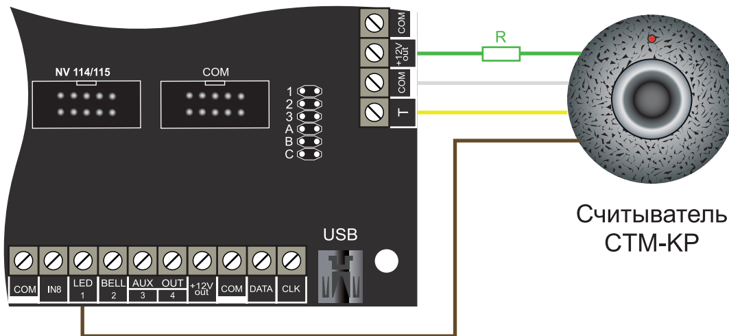
Рисунок 5. Схема подключения на примере ТМ считывателя СТМ-КТ
