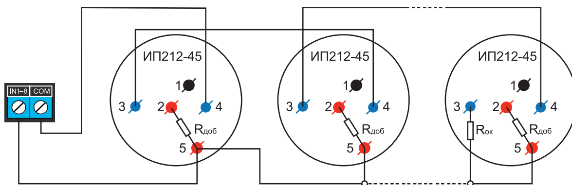
Рисунок 2. Схема подключения ИП212-45 к пожарному входу NV 8804 с добавочными и с окончечными резисторами
