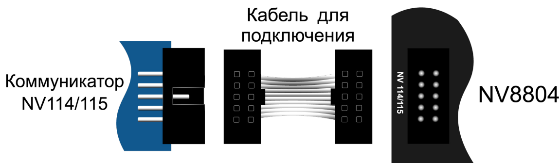
Рисунок 6. Подключение Ethernet/Wi-Fi к NV 8804
