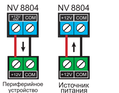
Рисунок 1. Подключение питания
