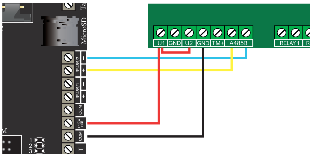
Рисунок 7. Подключение модуля Астра-РИ-М РР к NV 8804
