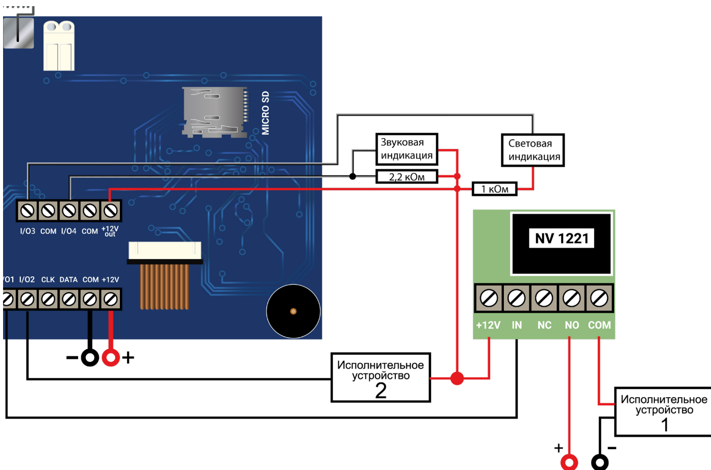
Рисунок 4. Пример подключения исполнительных устройств
