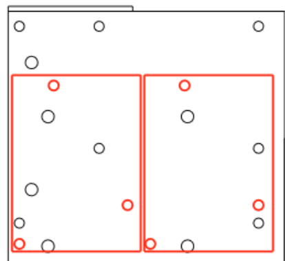
Расположение расширителей NV 2124
