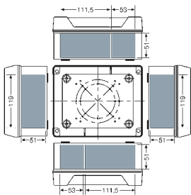
Стенки корпуса
