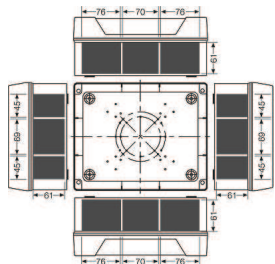
Стенки корпуса
