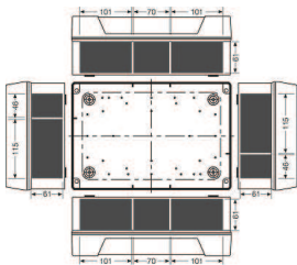
Стенки корпуса
