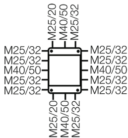
Чертеж с размерами
