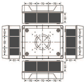
Стенки корпуса
