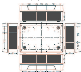
Стенки корпуса
