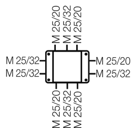
Стенки корпуса
