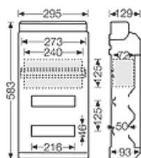
Чертеж с размерами
