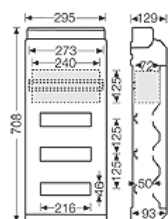
Чертеж с размерами
