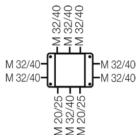
Стенки корпуса
