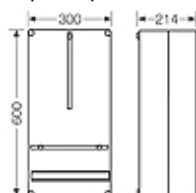
Чертеж с размерами
