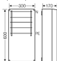
Чертеж с размерами
