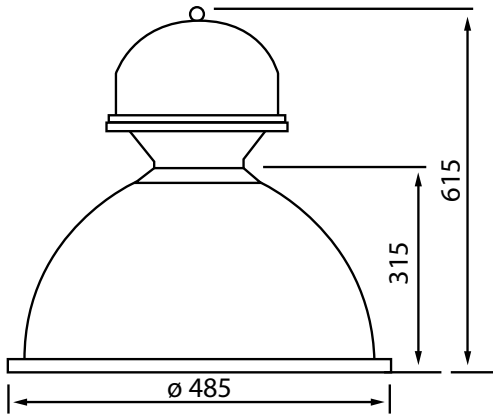
Схема светильника
