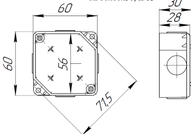
Основание КР60х60х30, IP65
