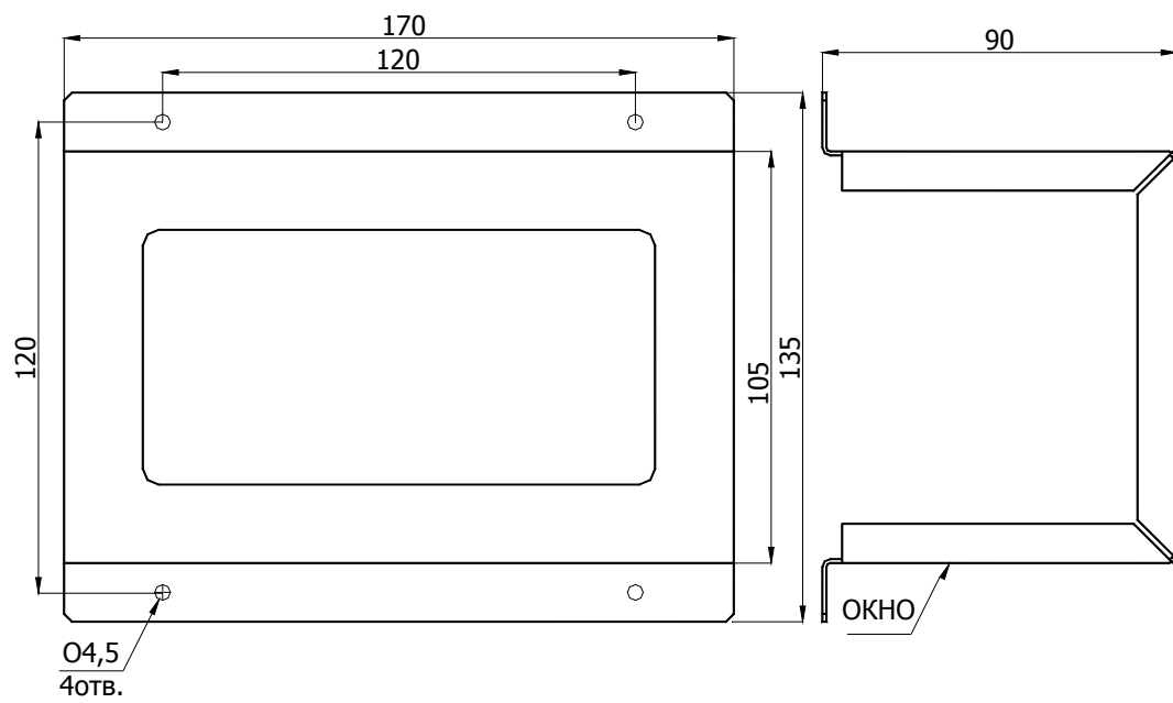
Рисунок 1 Общий вид кожуха
