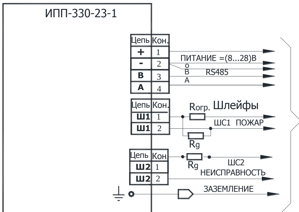
Рисунок 3 Схема подключения извещателя двумя шлейфами сигнализации с питанием шлейфов постоянным напряжением. Полярность шлейфов не соблюдается.
