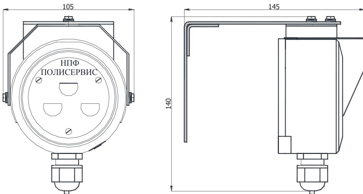
Рисунок 1 Общий вид извещателя
