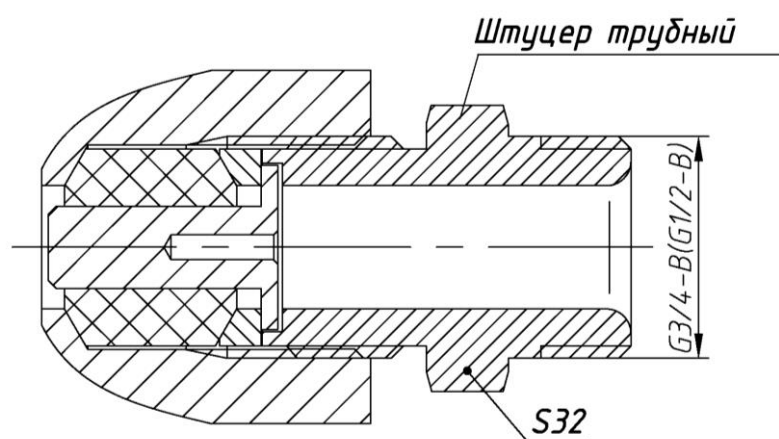
Рисунок А.4 Элементы кабельного ввода для прокладки кабеля в трубе. Остальное см. рисунок А.3
