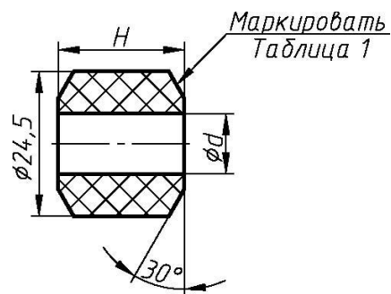
Рис .А.6 Кольцо уплотнительное в свободном состоянии. Переменные размеры приведены в таблице А.1
