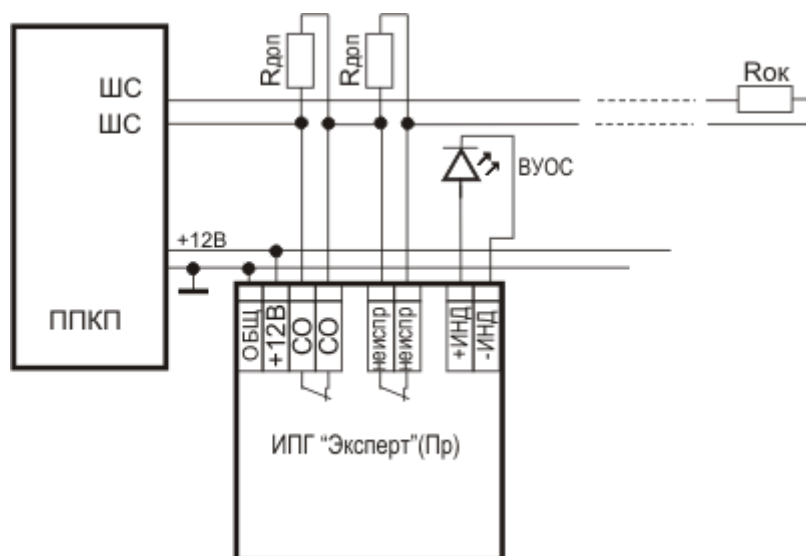
Рис.А.6. - Схема подключения ИП435-5 «Эксперт»(Пр) к ППКП (положение контактов реле ИП показаны в дежурном режиме) с объединением зон в один ШС. Величина резисторов R_{доп} и R_{ок} определяется в соответствии с техническим описанием ПКП. ВУОС – красный светодиод типа АЛ307.
