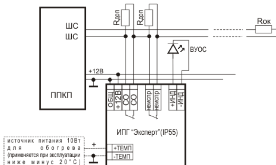
Рис.А.4. - Схема подключения ИП435-5 «Эксперт»(IP55) к ППКП (положение контактов реле ИП показаны в дежурном режиме) с объединением зон в один ШС. Величина резисторов R_{доп} и R_{ок} определяется в соответствии с техническим описанием ПКП. ВУОС – красный светодиод типа АЛ307.
