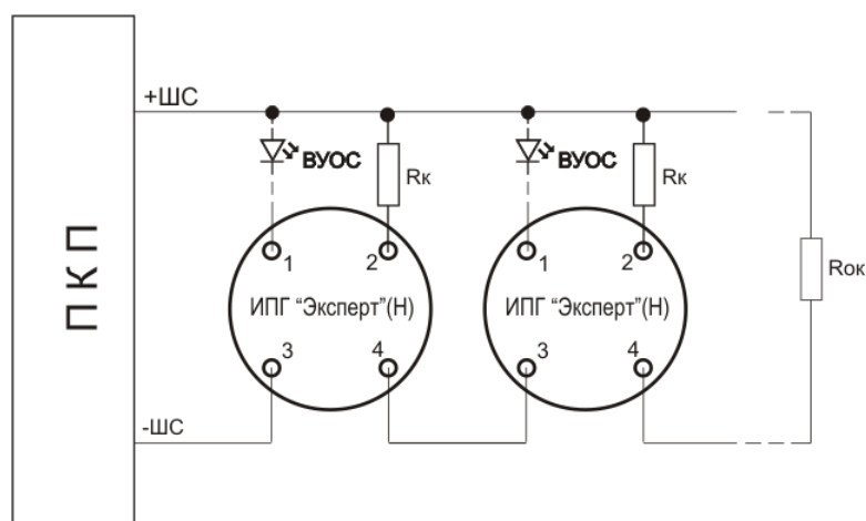
Рис.А.2. – Типовая схема включения извещателя ИП435-5 «Эксперт»(Н) к ПКП с однополярным шлейфом сигнализации. Величина резисторов Rк и Rок определяется в соответствии с техническим описанием ПКП. ВУОС – красный светодиод типа АЛ307.
