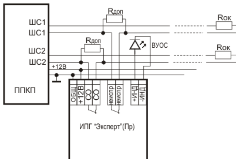
Рис.А.5. - Схема подключения ИП435-5 «Эксперт»(Пр) к ППКП (положение контактов реле ИП показаны в дежурном режиме) с включением зон в разные ШС. Величина резисторов R_{доп} и R_{ок} определяется в соответствии с техническим описанием ПКП. ВУОС – красный светодиод типа АЛ307.
