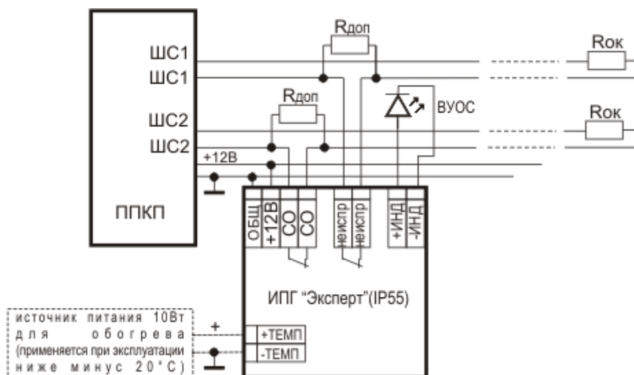
Рис.А.3. - Схема подключения ИП435-5 «Эксперт»(IP55) к ПКП (положение контактов реле ИП показаны в дежурном режиме) с включением зон в разные ШС. Величина резисторов Rдоп и Rок определяется в соответствии с техническим описанием ПКП. ВУОС – красный светодиод типа АЛ307.
