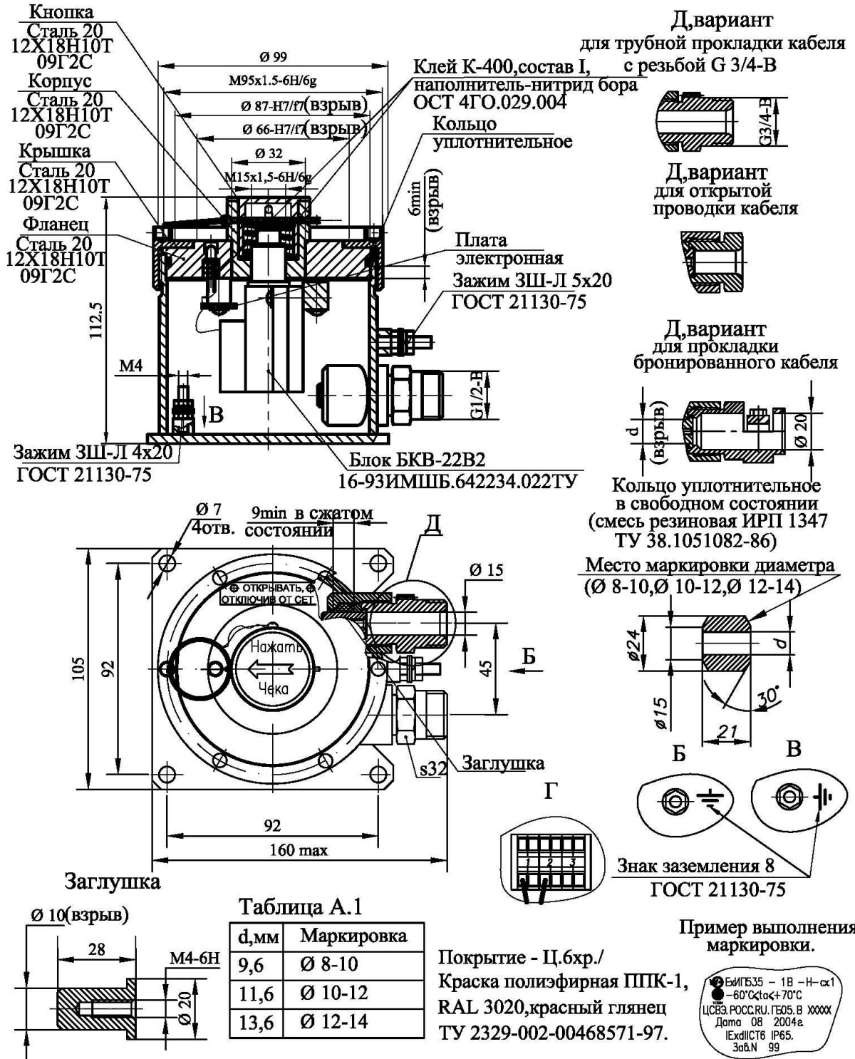
Рис. А.1 Габаритный чертеж извещателя Ех ИП535-1В в стальном корпусе, совмещённый с чертежом взрывозащиты
