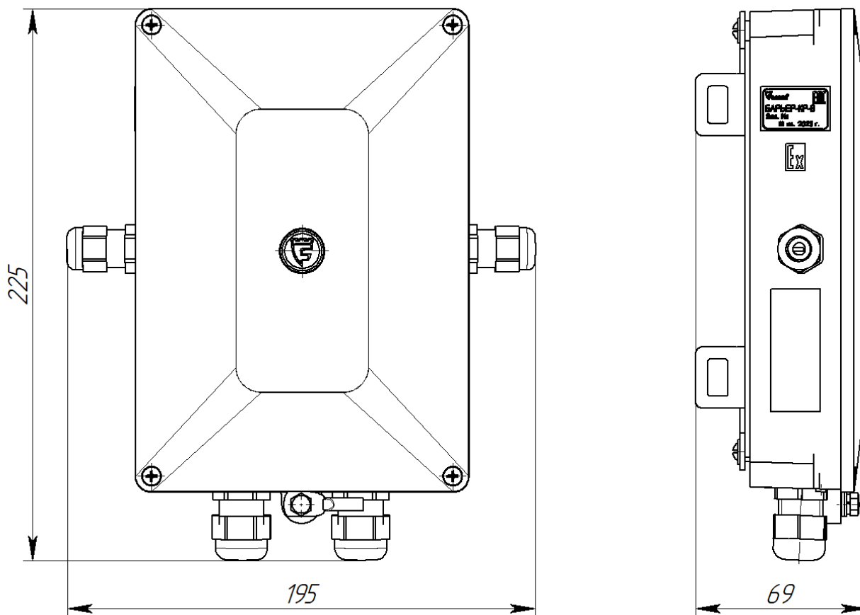
Рисунок 1 – Внешний вид коробки распределительной «БАРЬЕР-КР-В» ФРСБ.468344.012
