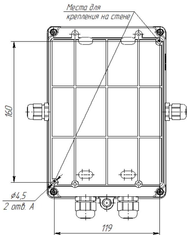
Рисунок 3 – Крепление коробки распределительной БАРЬЕР-КР-Б ФРСБ.468344.009 на стене
