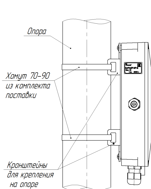
Рисунок 1 – Внешний вид коробки распределительной БАРЬЕР-КР-Б ФРСБ.468344.009
