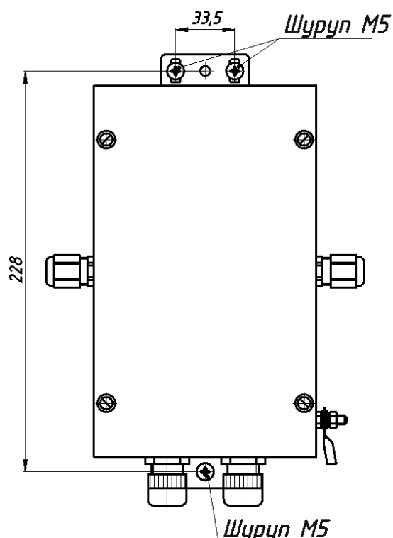
Рисунок 3 – Крепление коробки распределительной «БАРЬЕР-КР-В» ФРСБ.468344.004 на стене
