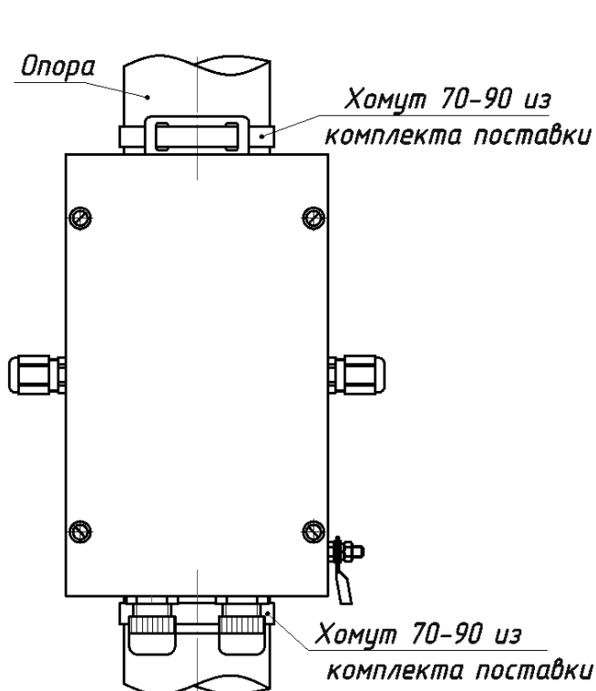
Рисунок 2 – Крепление коробки распределительной «БАРЬЕР-КР-В» ФРСБ.468344.004 на опоре
