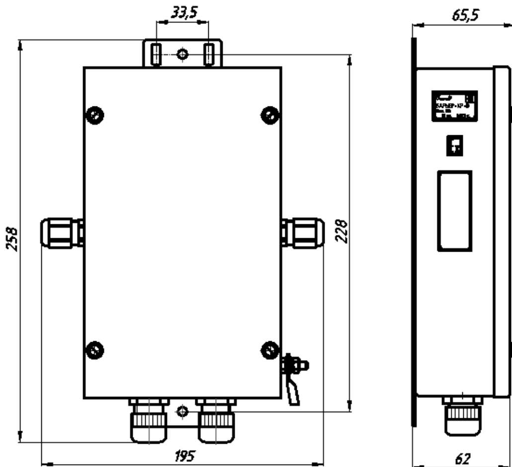
Рисунок 1 – Внешний вид коробки распределительной «БАРЬЕР-КР-В» ФРСБ.468344.004
