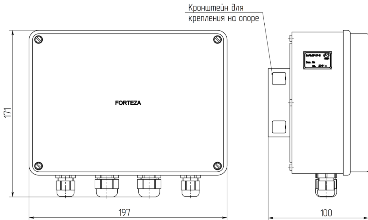
Рисунок 1 – Внешний вид коробки распределительной БАРЬЕР-KP-B ФРСБ.468344.003 для крепления на опоре
