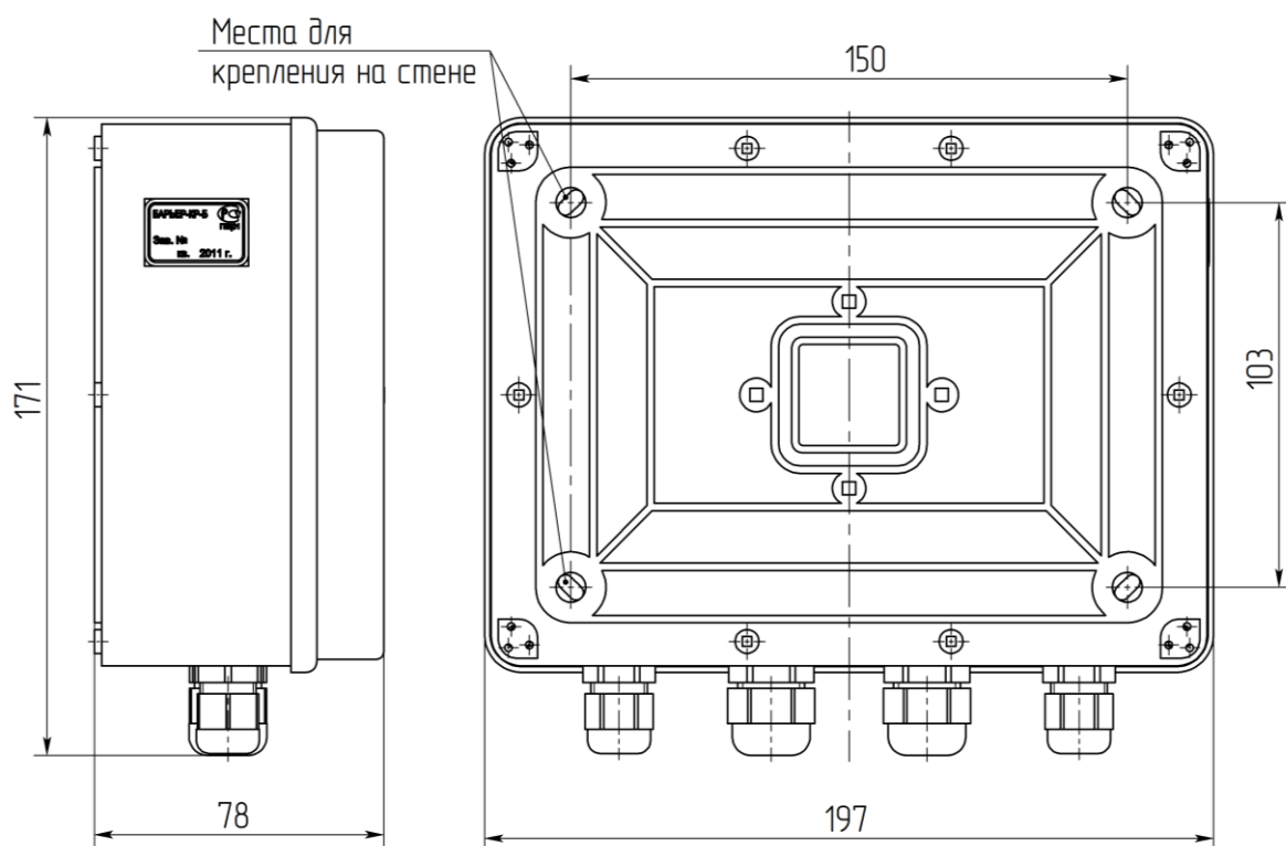
Рисунок 2 – Внешний вид коробки распределительной БАРЬЕР-KP-B ФРСБ.468344.003 для крепления на стене
