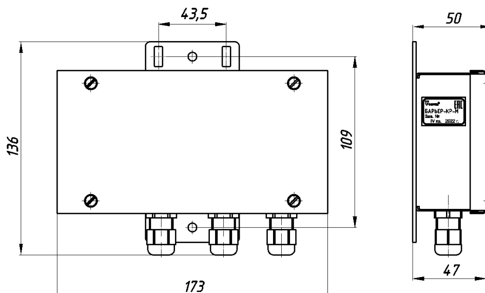
Рисунок 1 – Внешний вид коробки распределительной БАРЬЕР-КР-М ФРСБ.468344.007
