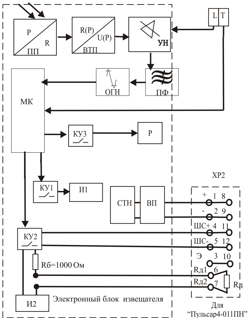
Рис 3 Схема функциональная
