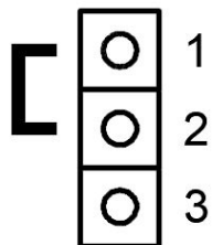
Рисунок 9 – Установка джампера согласующего резистора Переключатель в положении «1-2» – согласующий резистор подключен . Переключатель в положении «2-3» – согласующий резистор отключен .
