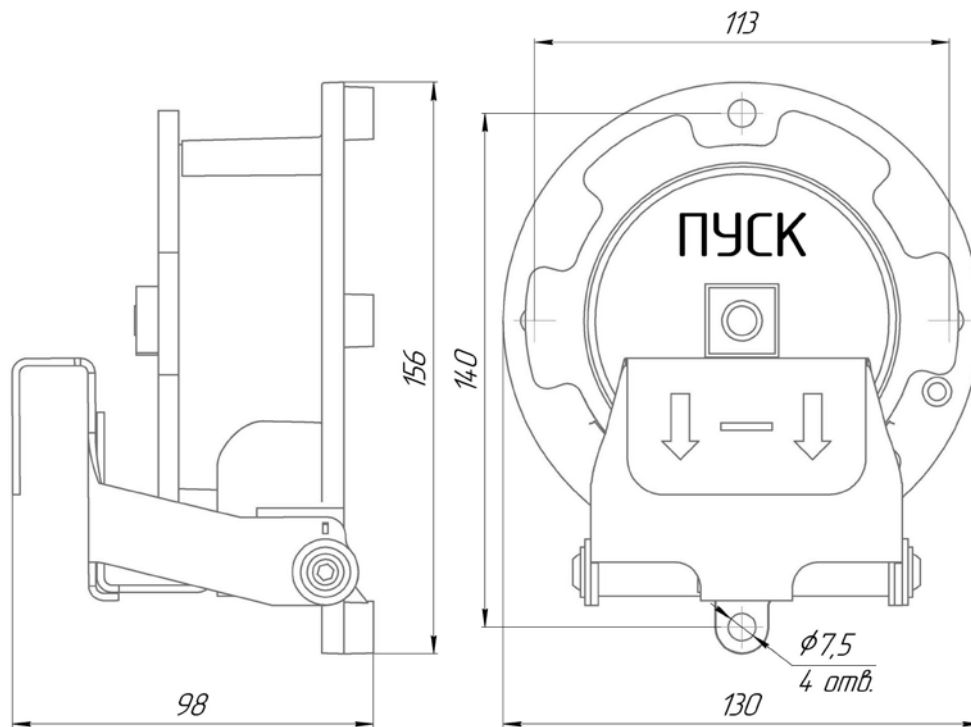
Рисунок А1 – Габаритные размеры УДП в алюминиевом корпусе
