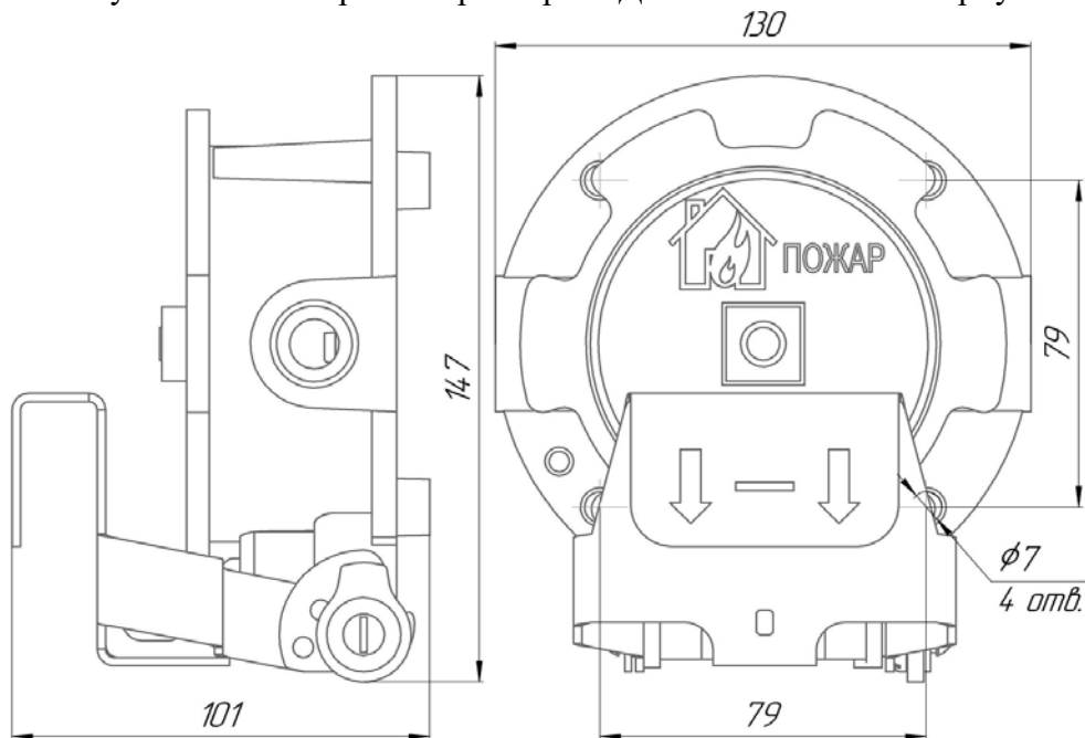
Рисунок А2 – Габаритные размеры УДП в нержавеющей корпусе
