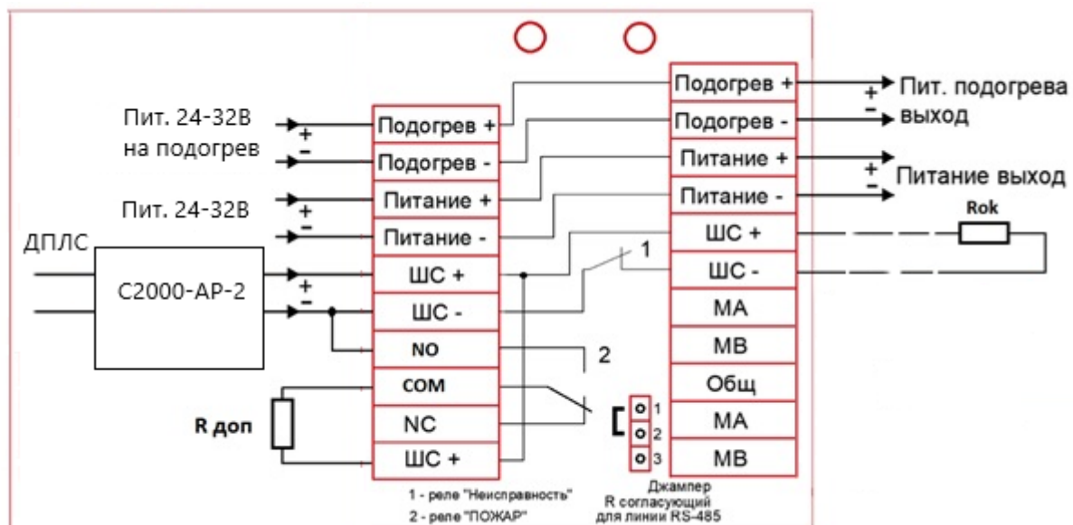
Рисунок 13 – Схема подключения с использованием C2000-AP-2
