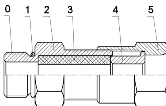
КВH – для монтажа открытого кабеля
