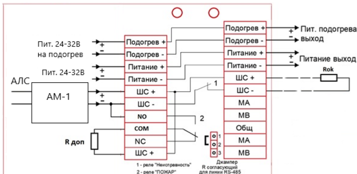
Рисунок 14 – Схема подключения с использованием AM-1
