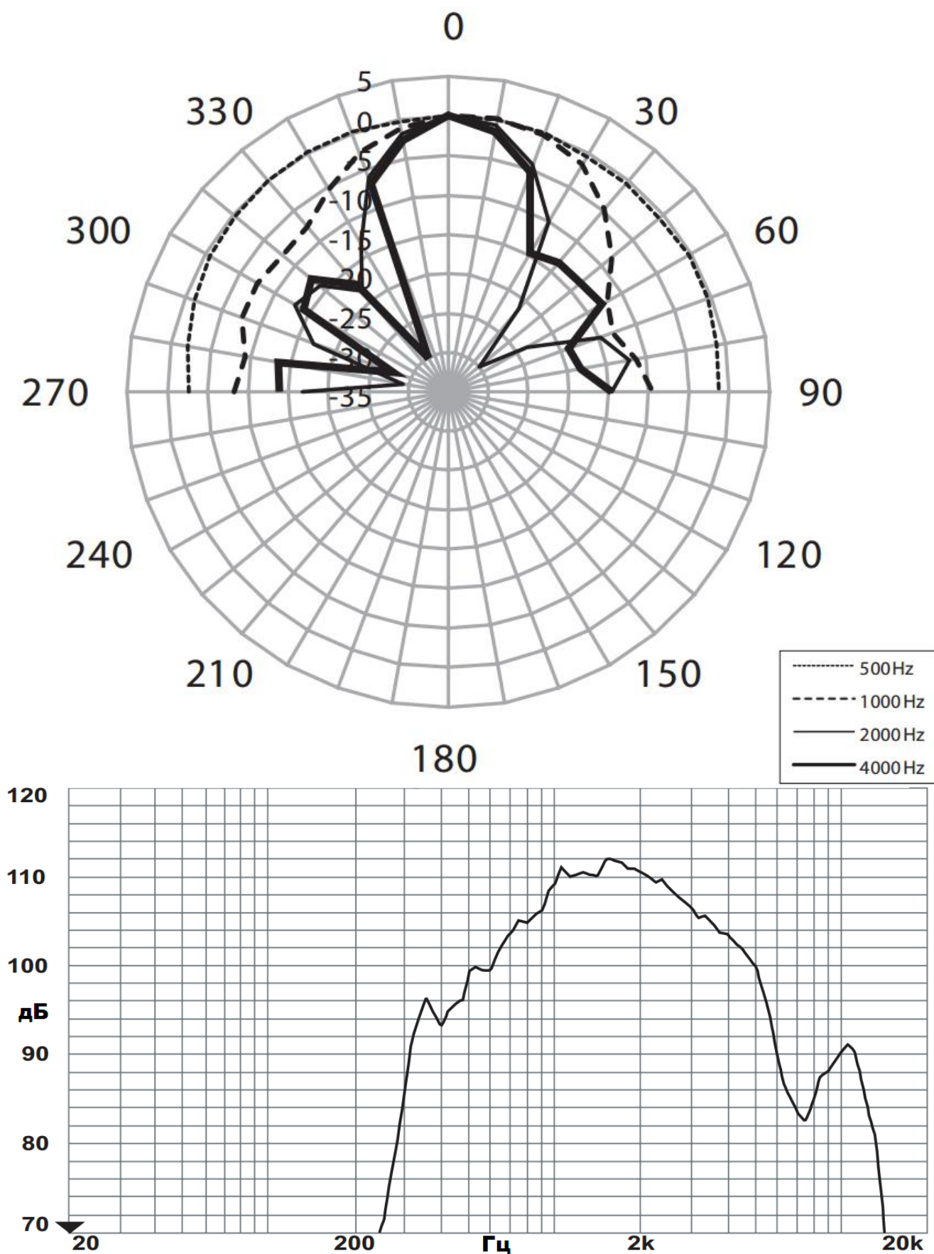
Рисунок 7 – Диаграмма направленности и амплитудно-частотная характеристика ГВР-Exd-10, ГВР-Exd-20
