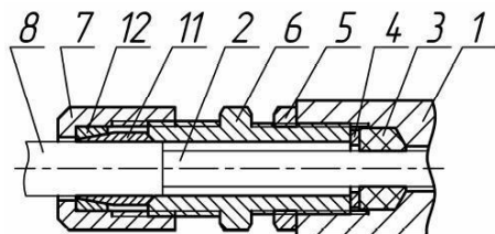
монтаж кабелем в металлорукове KB12 или бронированным кабелем
