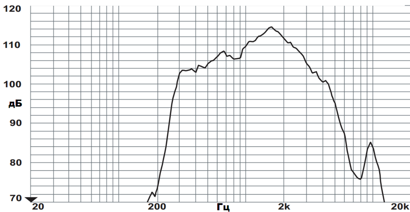
Рисунок 9 – Диаграмма направленности и амплитудно-частотная характеристика ГВР-Exd-50
