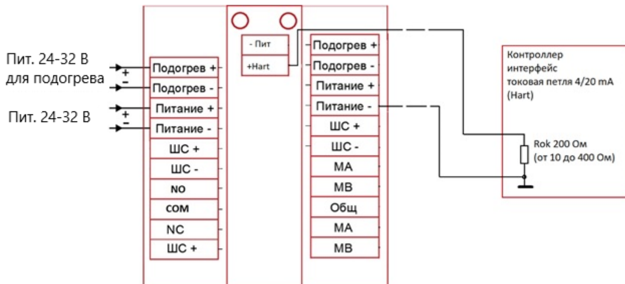
Рисунок 12 – Клеммная плата извещателя
