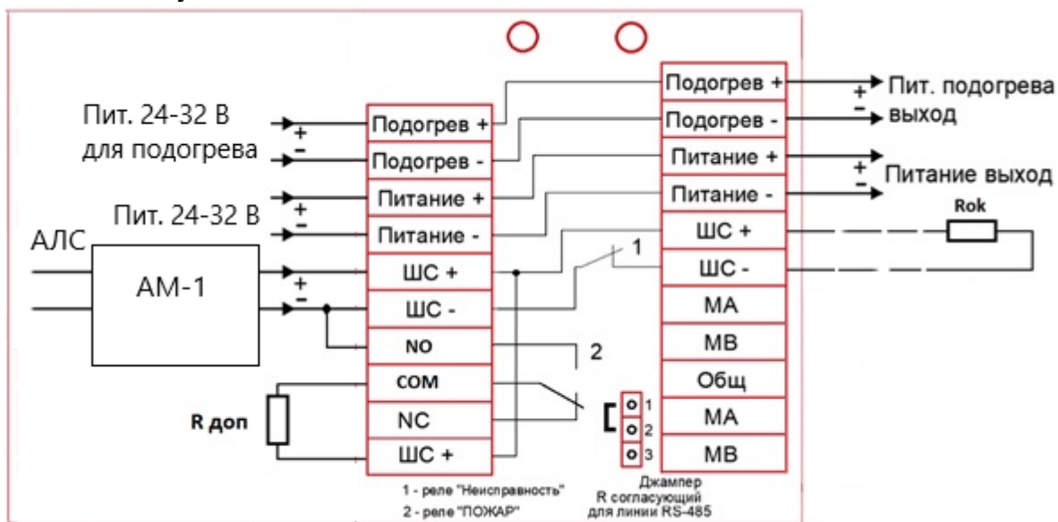
Рисунок 14 – Схема подключения с использованием АМ-1
