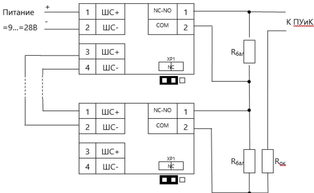
Рисунок А4. 4х-проводная схема подключения извещателя в шлейф сигнализации. Только для извещателей в исп. СПЕТКРОН-535-(Ex)-ИПР-В исп. 01.
