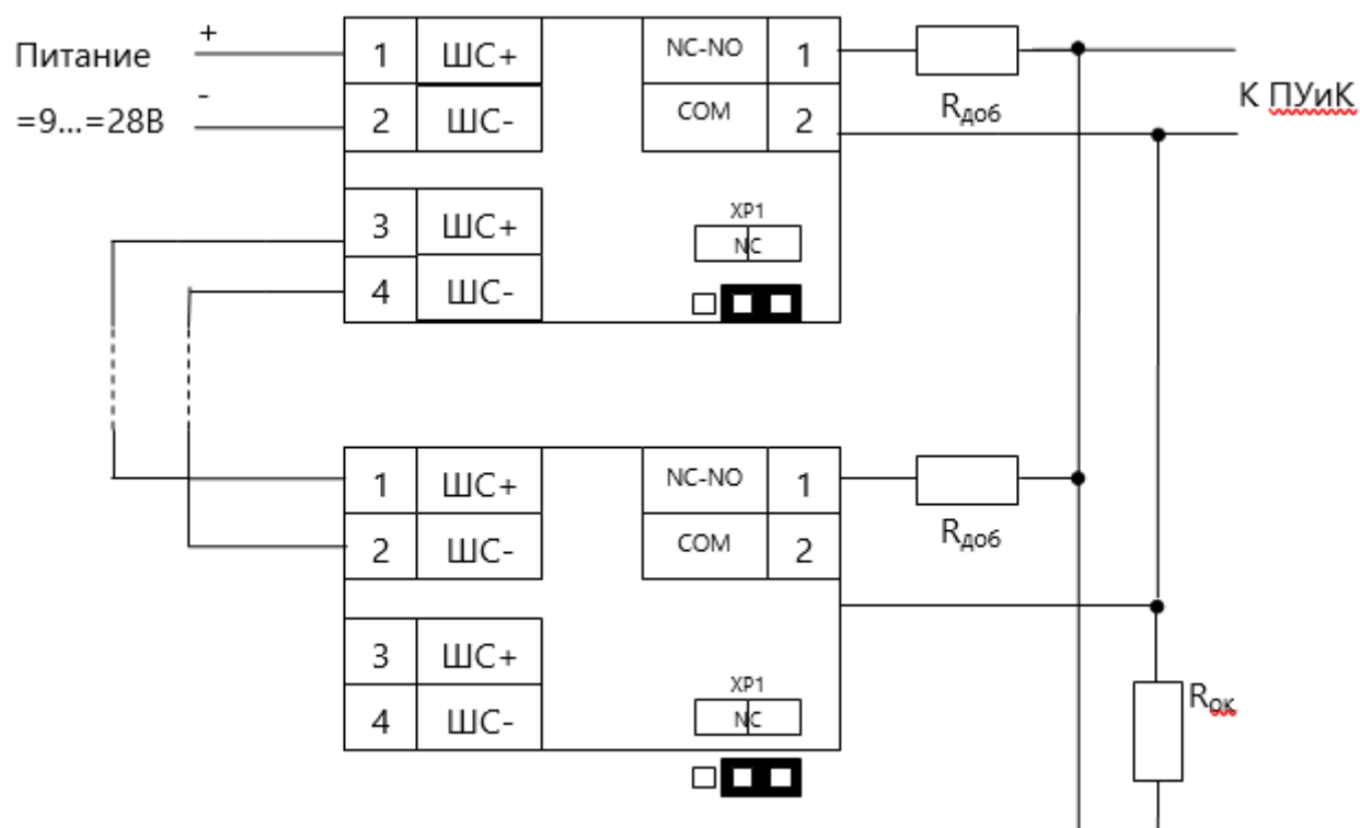
Рисунок А3. 4х-проводная схема подключения извещателя в шлейф сигнализации. Только для извещателей в исп. СПЕТКРОН-535-(Ex)-ИПР-В исп. 01.
